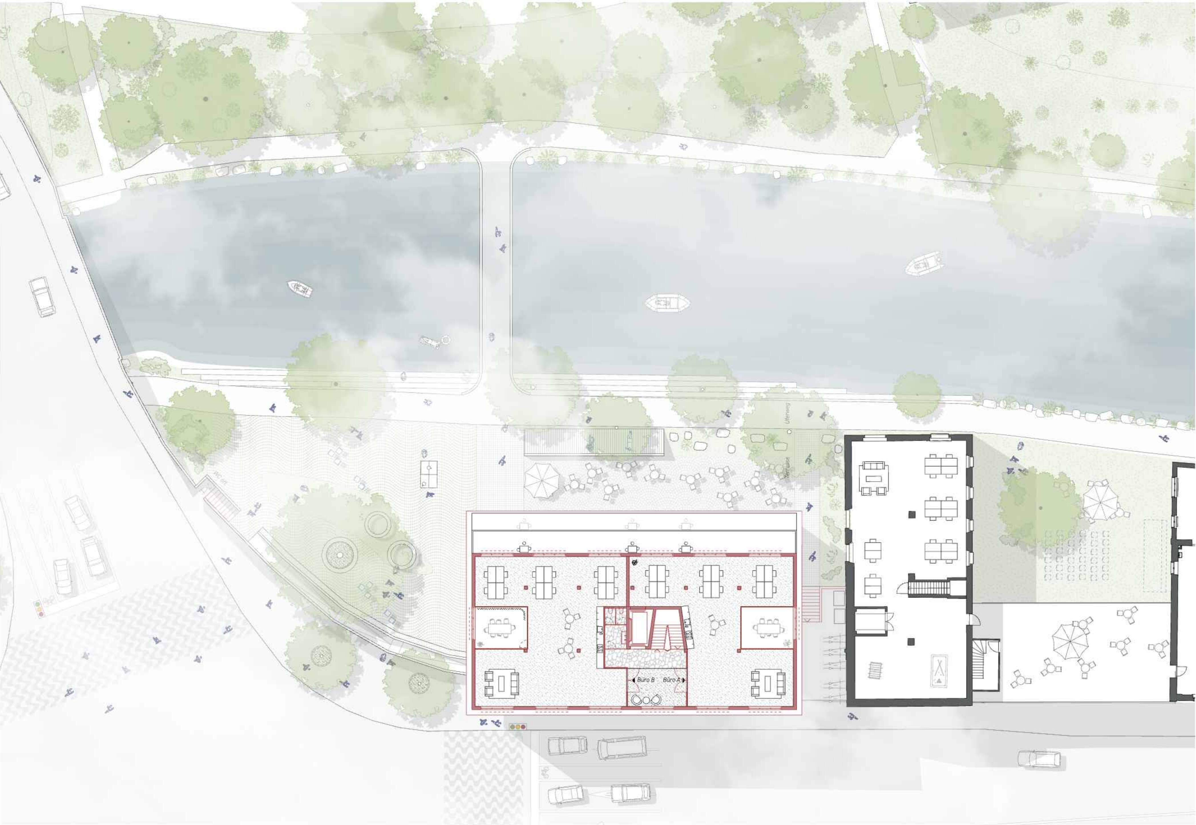
Grundriss 1, Obergeschoss 1:200
