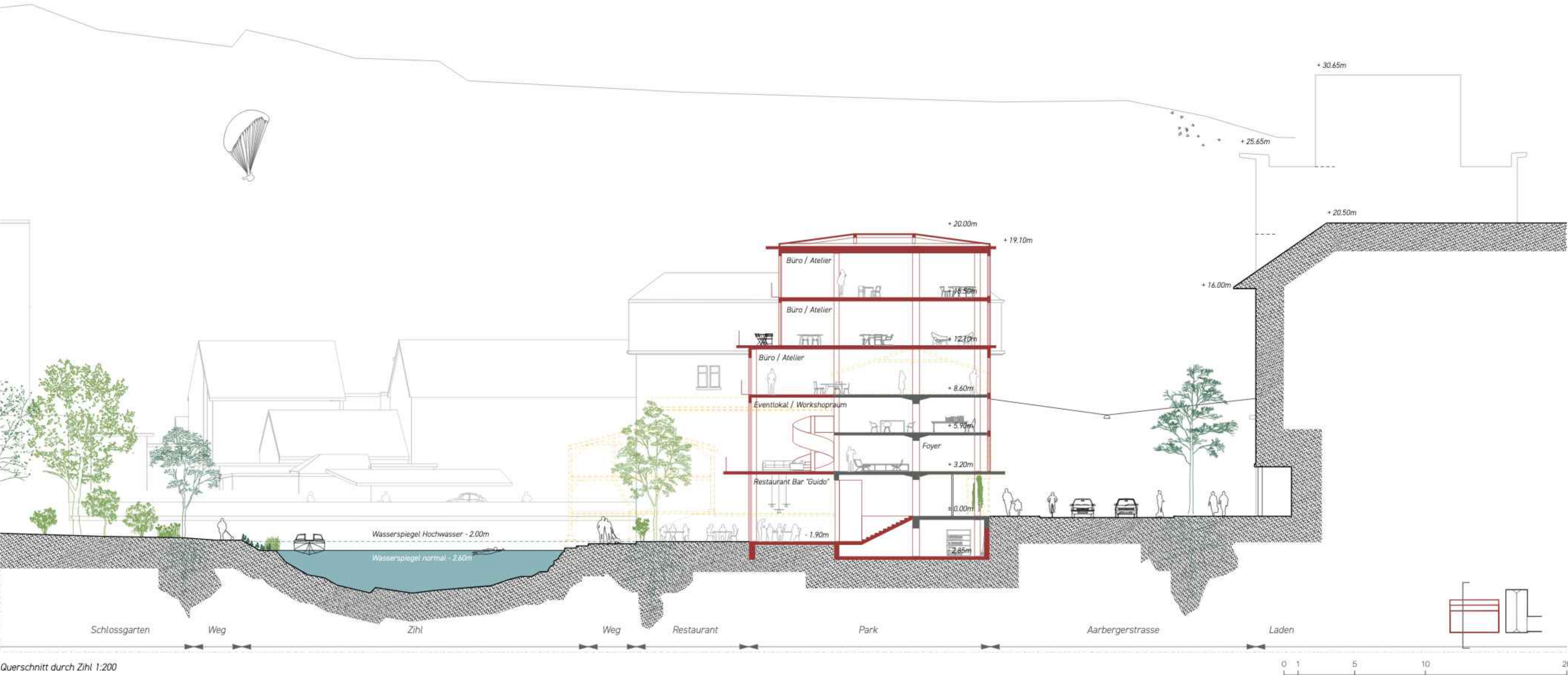
Querschnitt durch Zihl 1:200
