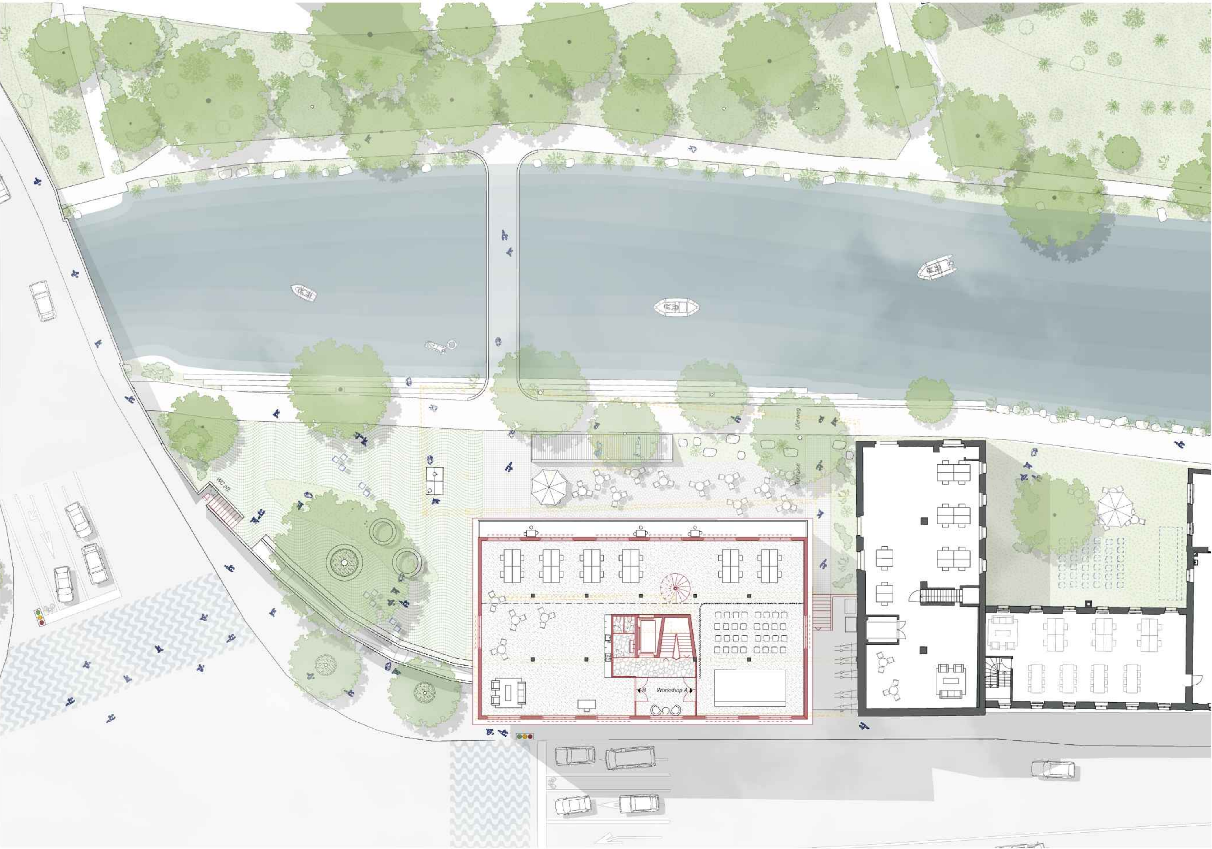
Grundriss 1, Obergeschoss 1:200
