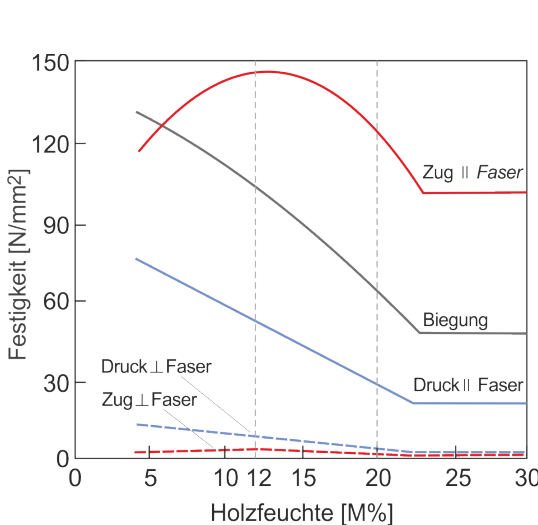
Abb. 1: Festigkeit von Holz in Abhängigkeit der Holzfeuchte, Kretschmann (2010)
