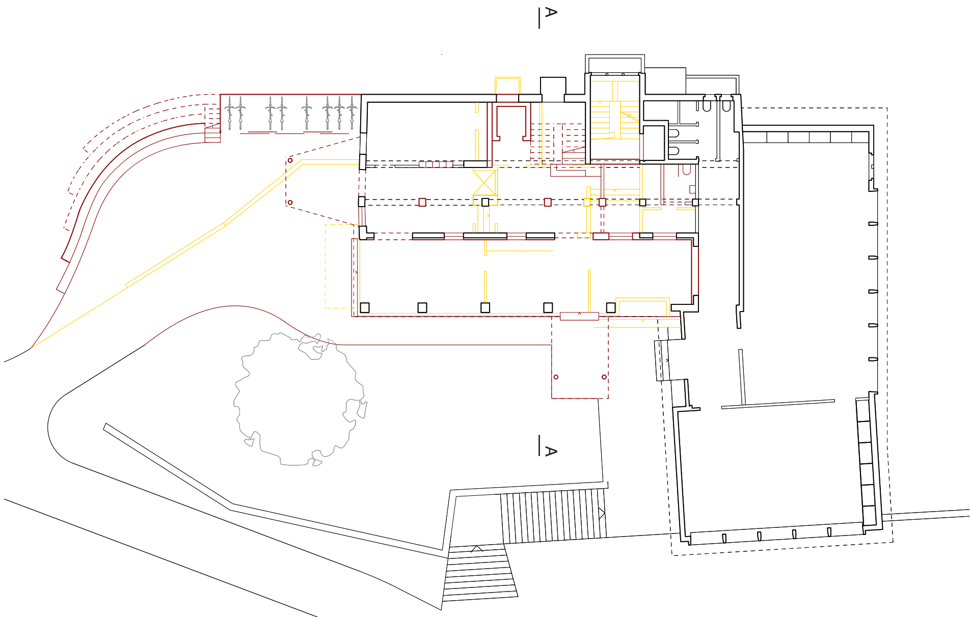
Grundriss Erdgeschoss | 1:200
