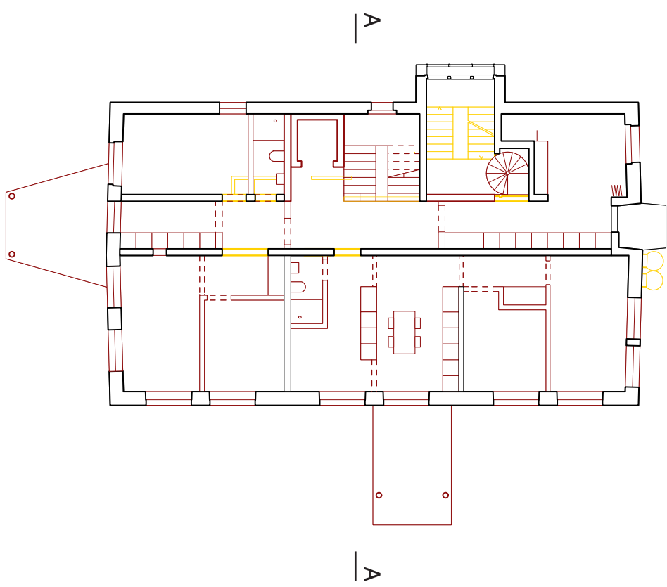
Grundriss 3. Geschoss | 1:200
