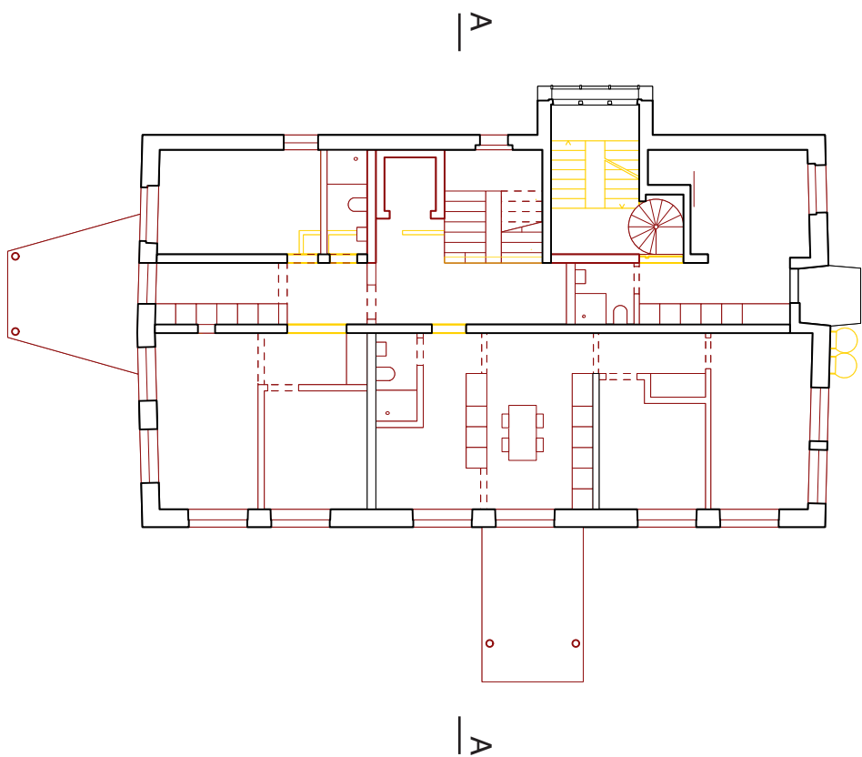
Grundriss 4. Geschoss | 1:200
