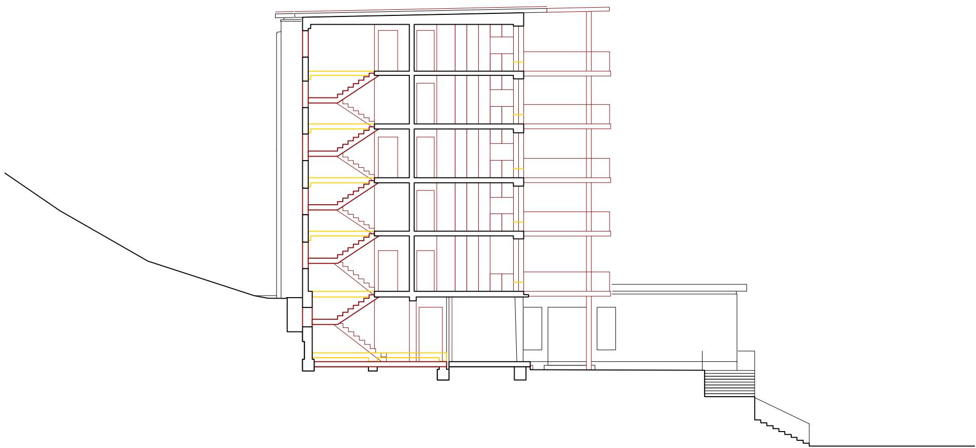
Schnitt AA | 1:200
