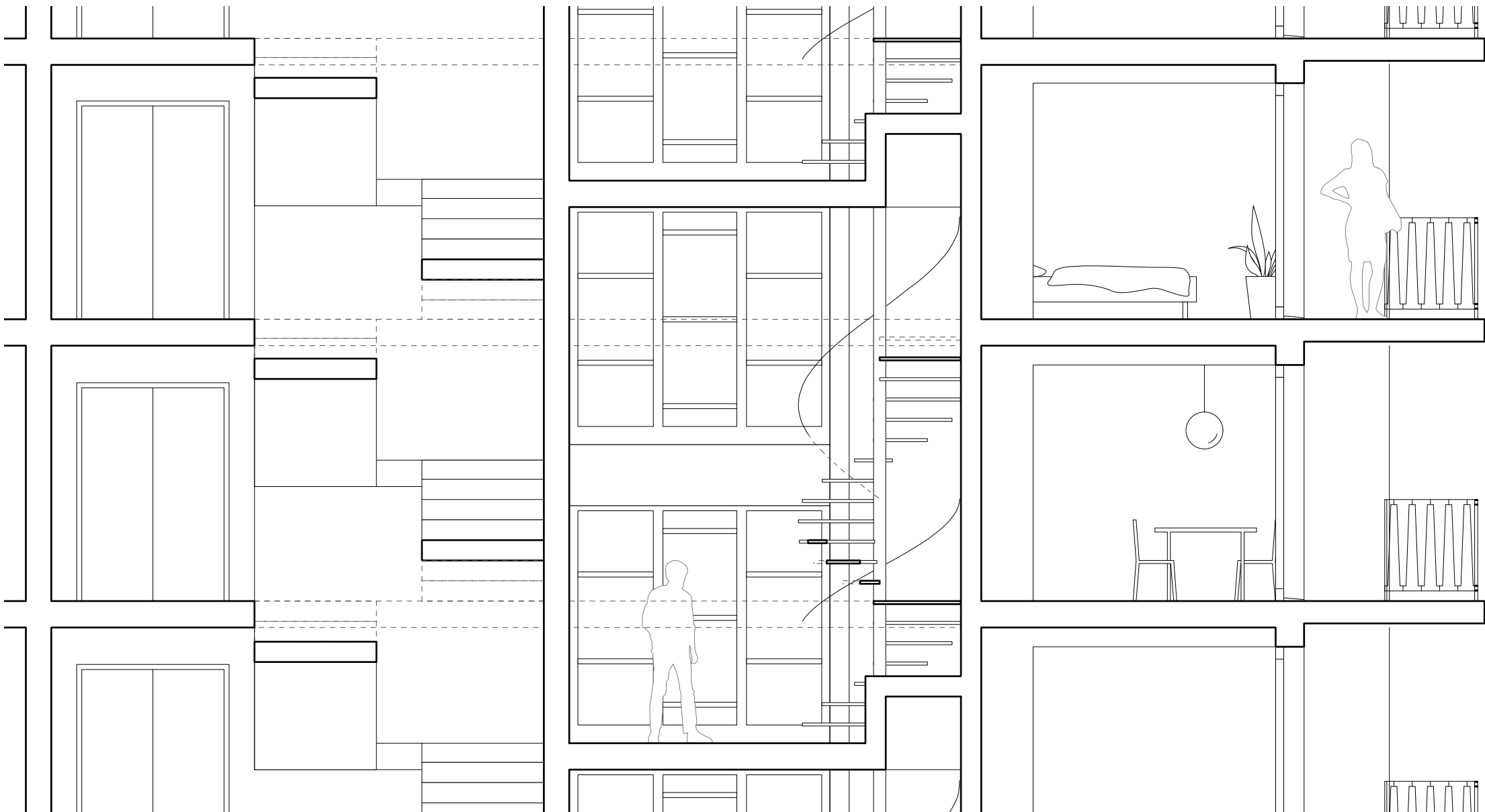
Wohnungsschnitt BB Maisonette I 1:50
