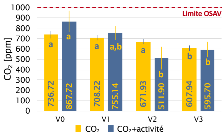
Graphique 1: Moyennes modélisées du CO 2 en fonction des variables de température et d'humidité relative, et comparaison avec la prise en compte de la variable de l'activité des chevaux.
