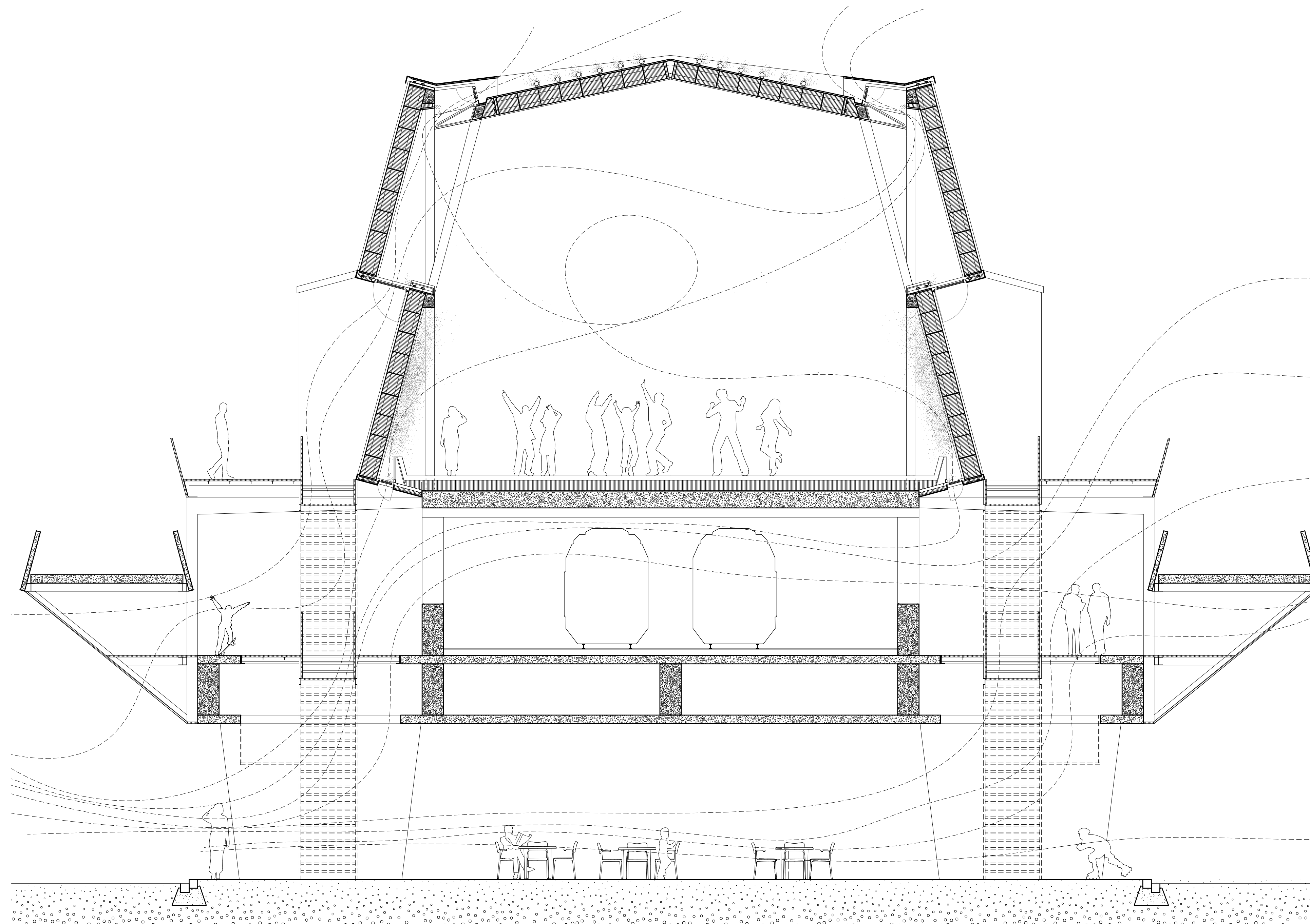
Emergenz und Obsoleszenz - Barn 1:60 Konstruktion Nick Christian Orin Fahrni Bachelor Thesis Frühling 2026
