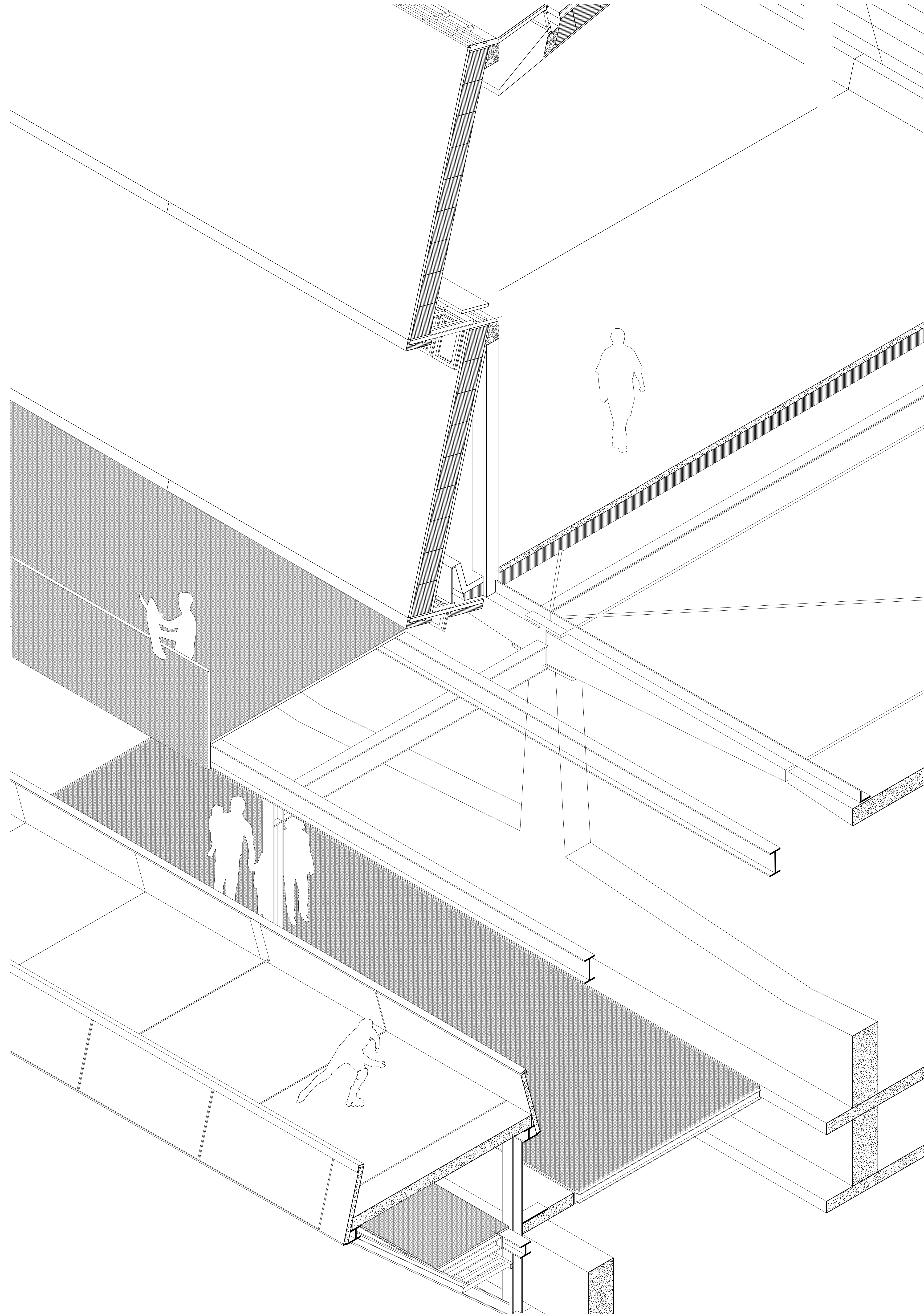
Emergenz und Obsoleszenz - Barn 1:25 Detail Konstruktion Nick Christian Orin Fahrni Bachelor Thesis Frühling 2026
