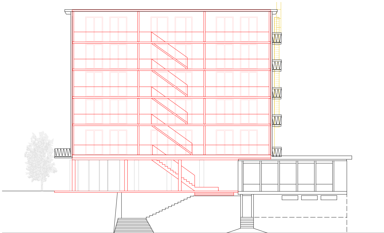
Südfassade, 1:200
