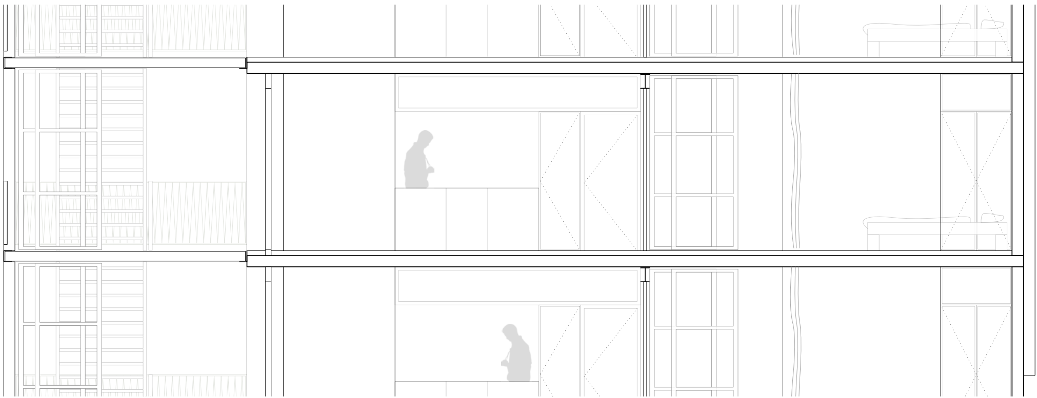
Wohnungsschnitt, 1:50
