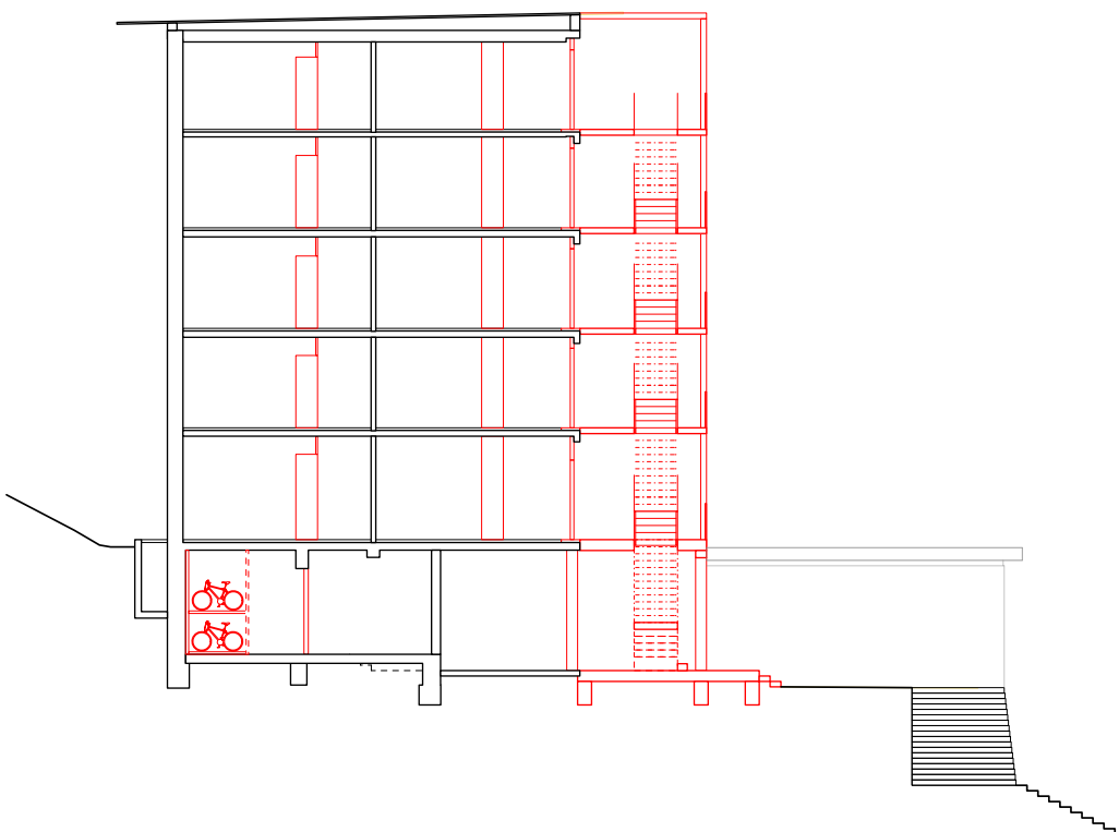
Schnitt, 1:200
