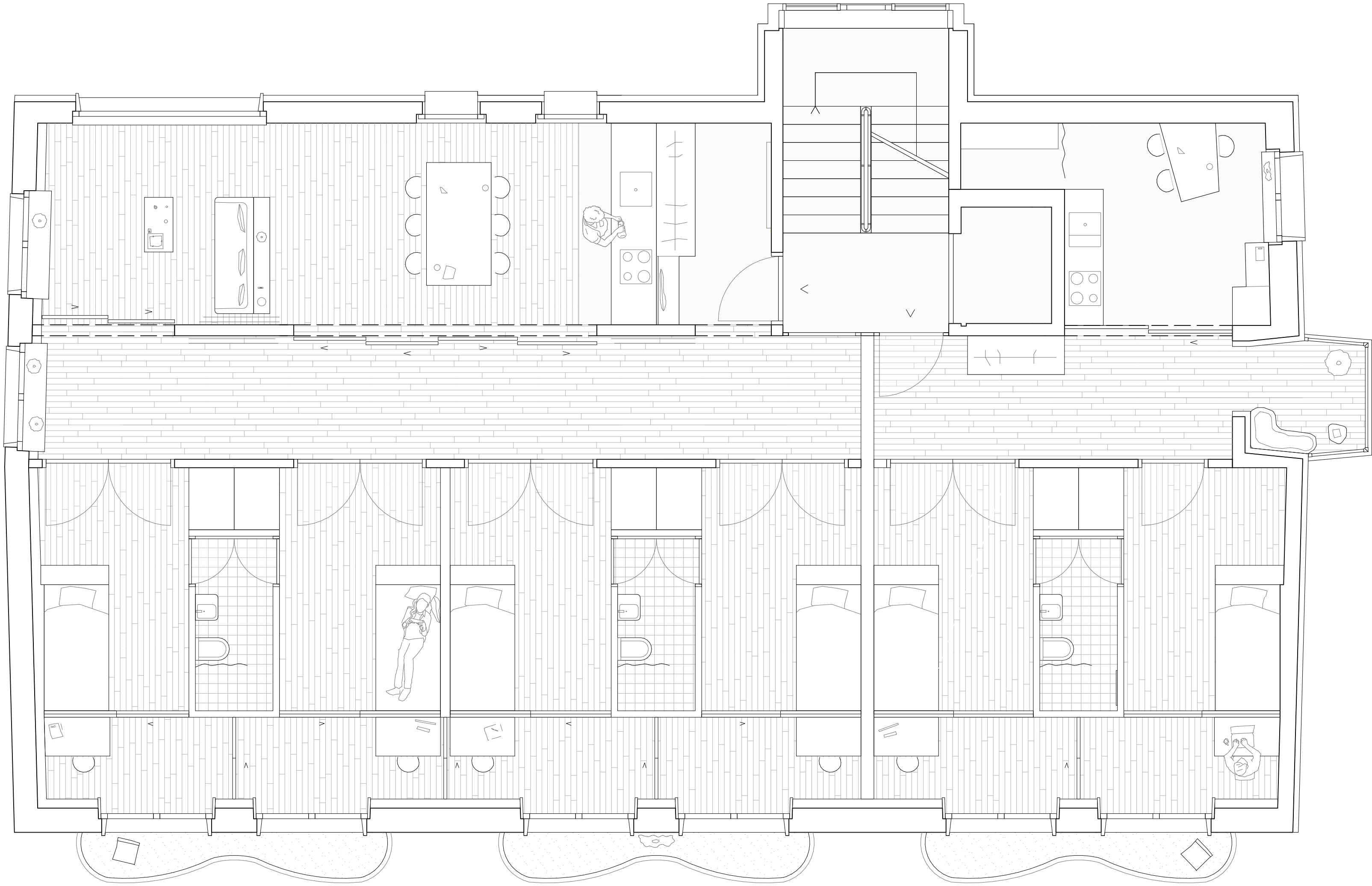
Grundriss Wohnung
